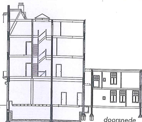
doorsnede
